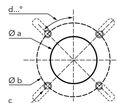
Brida de conexión
