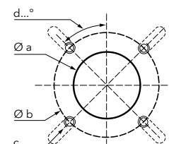
Brida de conexión
